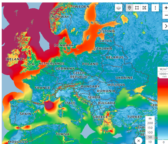
A2.2. ábra: Magyarország szélenergia-lehetőségeinek összehasonlítása más országokéval és régiókéval [A2.4].
