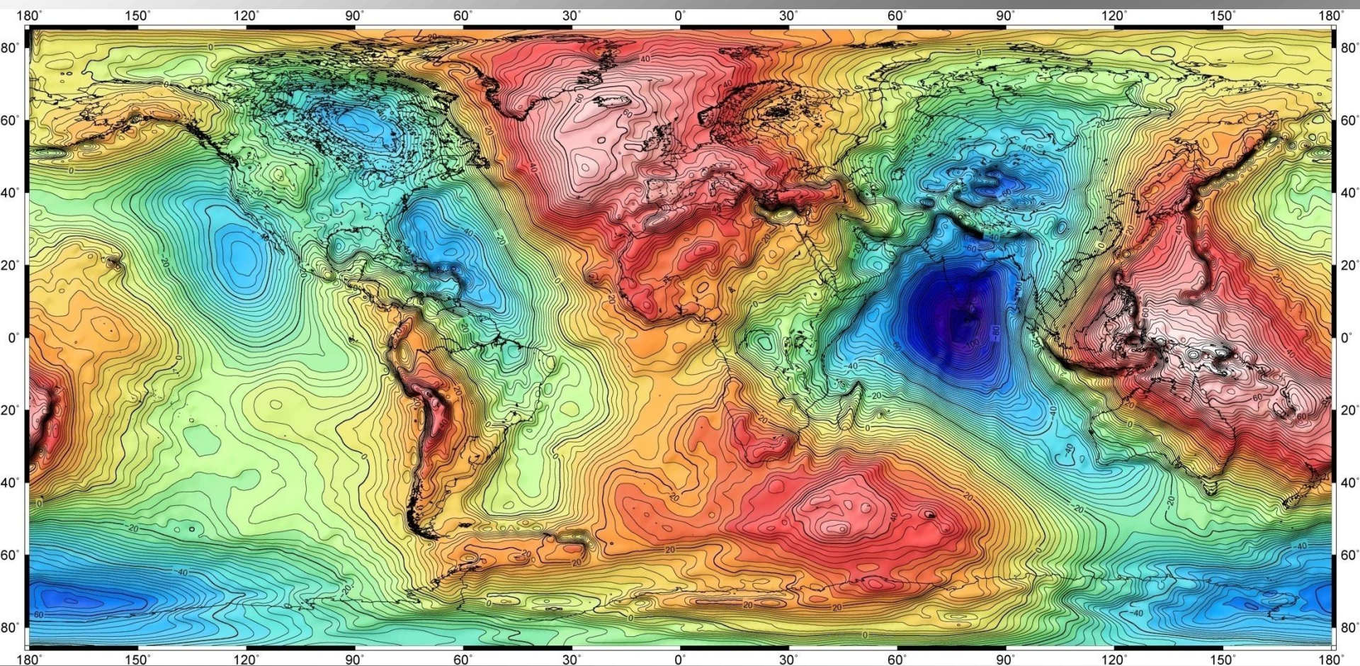
Az EGM2008 geopotenciál modellből számított geoidkép
